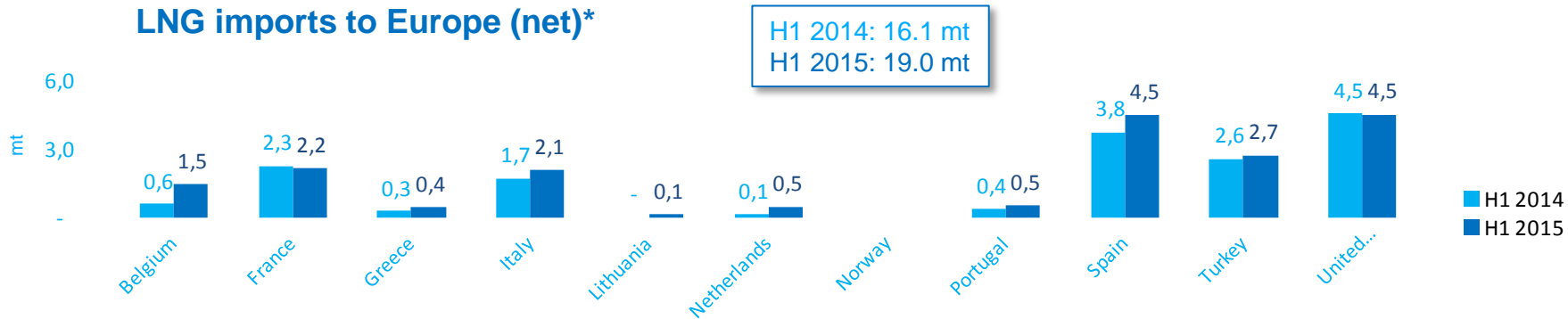
Origin of European LNG imports
